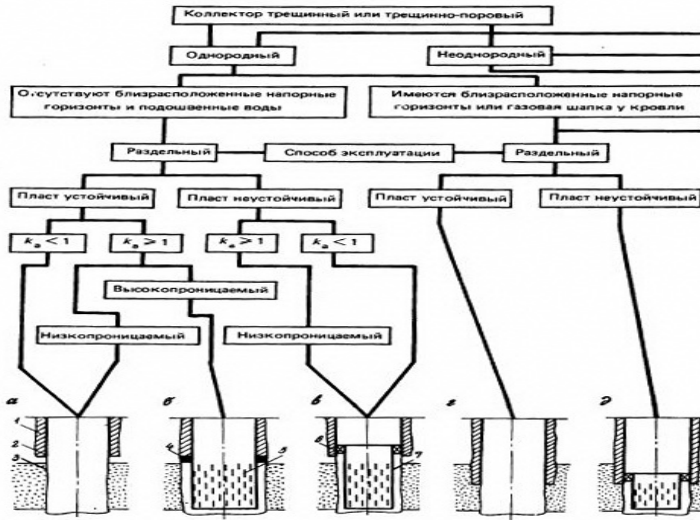
Рис. 1 Основные конструкции эксплуатационного забоя скважин и условия их применения: 3—открытый забой скважины; 4—пакер; 5—фильтр; 6—пакер; 7—потайная колонна-фильтр.
